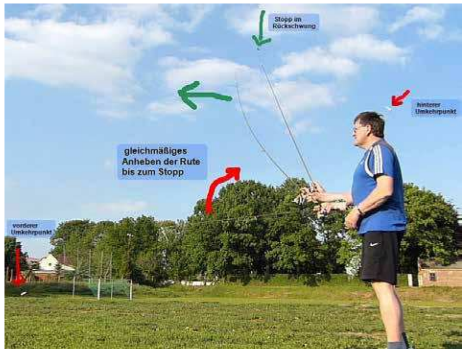
Bild 4: Vorschwing beim Rundwurf, einer Variante des Überkopfwurfes. (© K.-J. Bruder)
